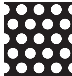
5φ×8P 開孔率（約35％）
