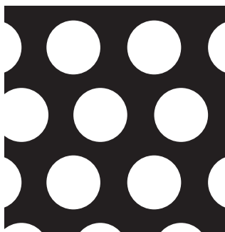
10φ×15P 開孔率（約40％）
