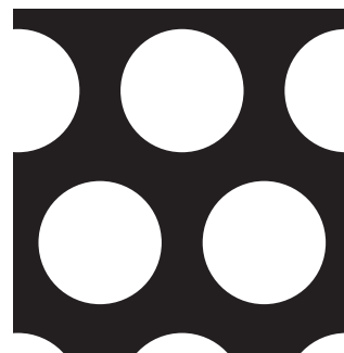
15φ×20P 開孔率（約51％）
